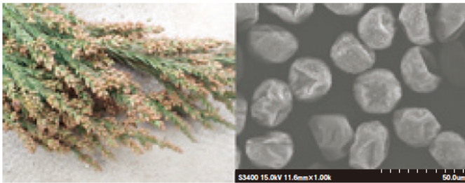
スギの雄花とスギ花粉の電子顕微鏡写真（1000倍）
